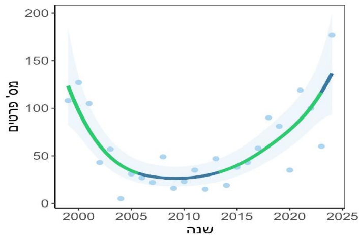
איור 9 – מגמות השינוי ארוכות הטווח בהרי אילת והערבה במודל GAMM הנקודות בתכלת – תוצאות הספירות, קו המגמה בכחול כהה – ללא שינויים מובהקים בין השנים בגודל האוכלוסייה, קו המגמה בירוק – שינויים מובהקים בין השנים בגודל האוכלוסייה.
