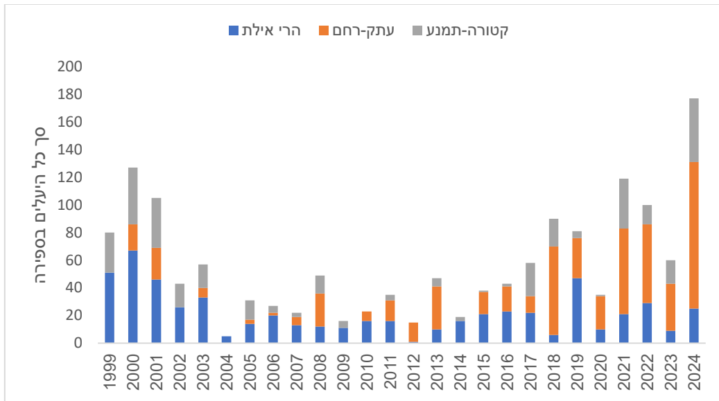
איור 10 – ספירות יעלים באילת לפי אזורי הספירה השונים: הר'י אילת, עתק-רחם וקטורה-תמנע
