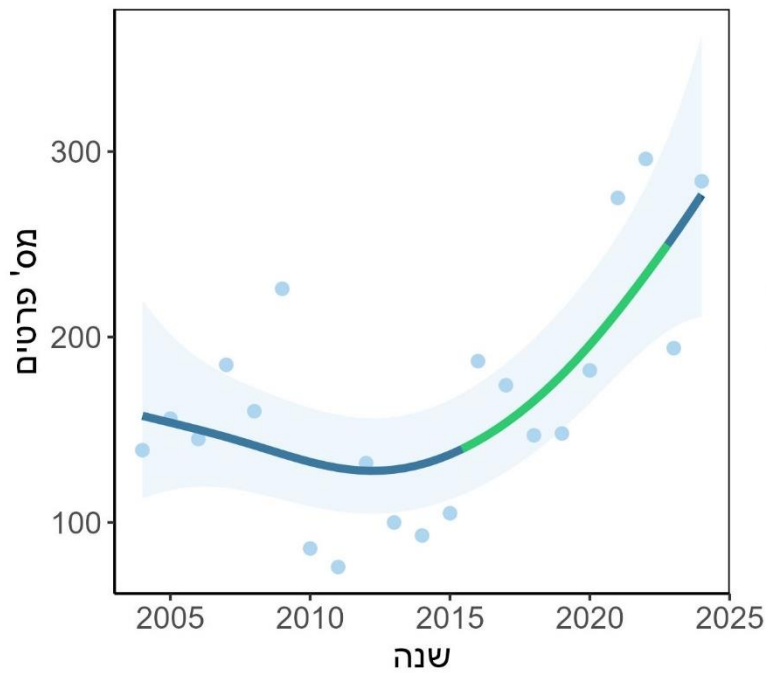
איור 3 – מגמות שינוי ארוכות הטווח בצפון מדבר יהודה במודל GAMM. הנקודות בתכלת – תוצאות הספירות, קו המגמה בכחול כהה – ללא שינויים מובהקים בגודל האוכלוסייה בין השנים, קו המגמה בירוק – שינויים מובהקים בגודל האוכלוסייה בין השנים.
