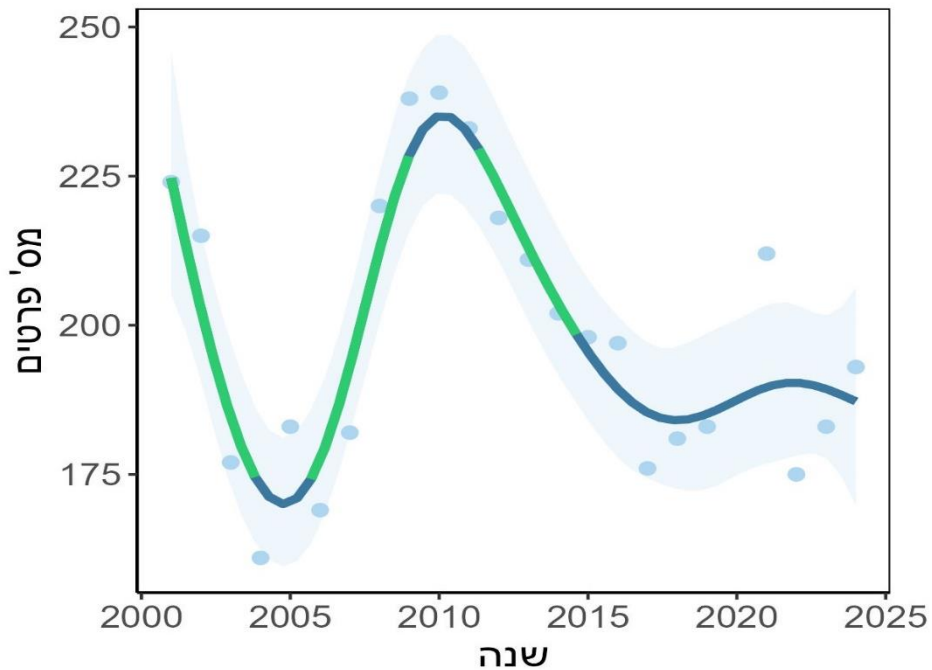
איור 5 – מגמות השינוי ארוכות הטווח בעין גדי במודל GAMM. הנקודות בתכלת – תוצאות הספירות, קו המגמה בכחול כהה – ללא שינויים מובהקים בין השנים בגודל האוכלוסייה, קו המגמה בירוק – שינויים מובהקים בין השנים בגודל האוכלוסייה.
