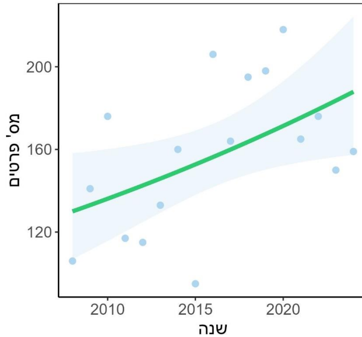
איור 6 – מגמות השינוי ארוכות הטווח בבקעת צין במודל GAMM. הנקודות בתכלת – תוצאות הספירות, קו המגמה בירוק – שינויים מובהקים בגודל האוכלוסייה בין השנים.
