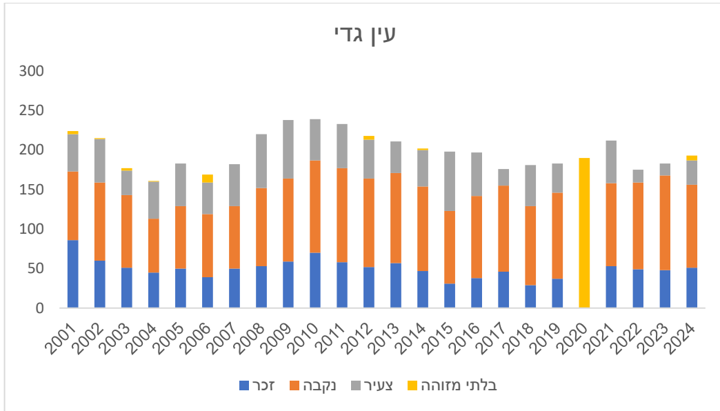
איור 4 – אוכלוסיית היעלים הכללית בעין גדי לפי שנים בחלוקה לזכרים, נקבות, צעירים ובלתי מזוהים. בשנת 2020 לא נעשתה ספירה ובגרף מוצגת תוצאה של השלמה ממודל.
