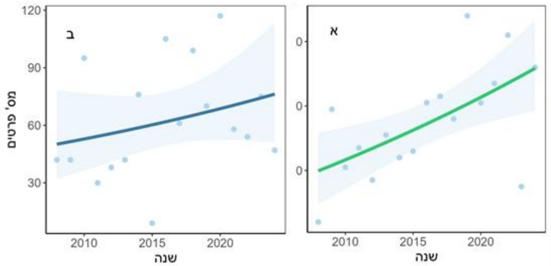
איור 8 – מגמות השינוי ארוכות הטווח בבקעת צין בשטח מיושב (א) לעומת בשטח טבעי (ב) במודל GAMM. הנקודות בתכלת – תוצאות הספירות, קו המגמה בכחול כהה – ללא שינויים מובהקים בין השנים בגודל אוכלוסייה, קו המגמה בירוק – שינויים מובהקים בין השנים בגודל האוכלוסייה.
