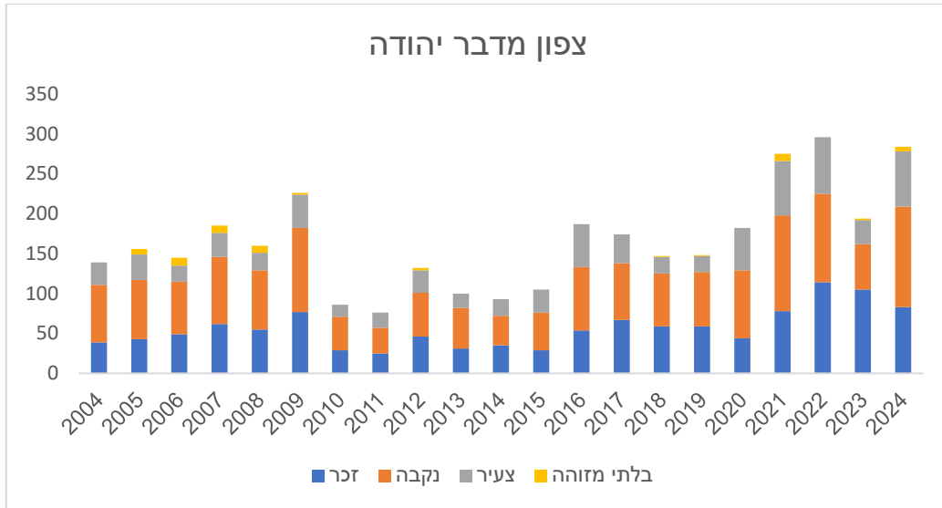
איור 2 – אוכלוסיית היעלים בצפון מדבר יהודה לפי שנים בחלוקה לזכרים, נקבות, צעירים ובלתי מזוהים
