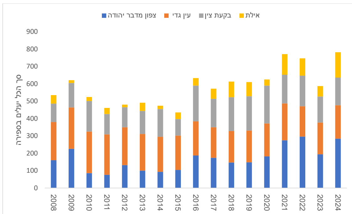
איור 1 – תוצאות הספירה של אוכלוסיית היעלים בכל אחד מאזורי הספירה
